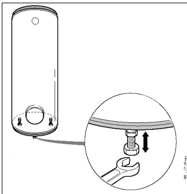
Рис. 4.4 Выравнивание водонагревателя
